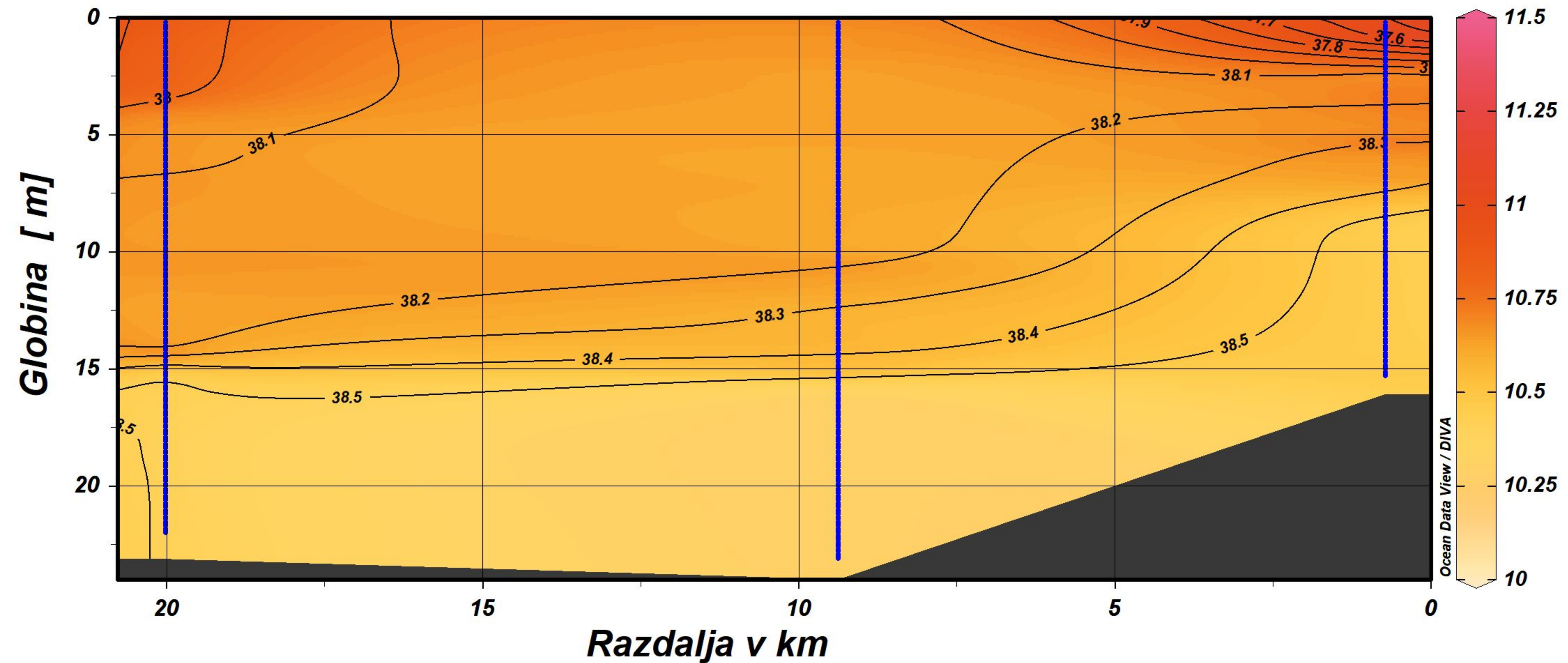
Temperatura [ °C]
