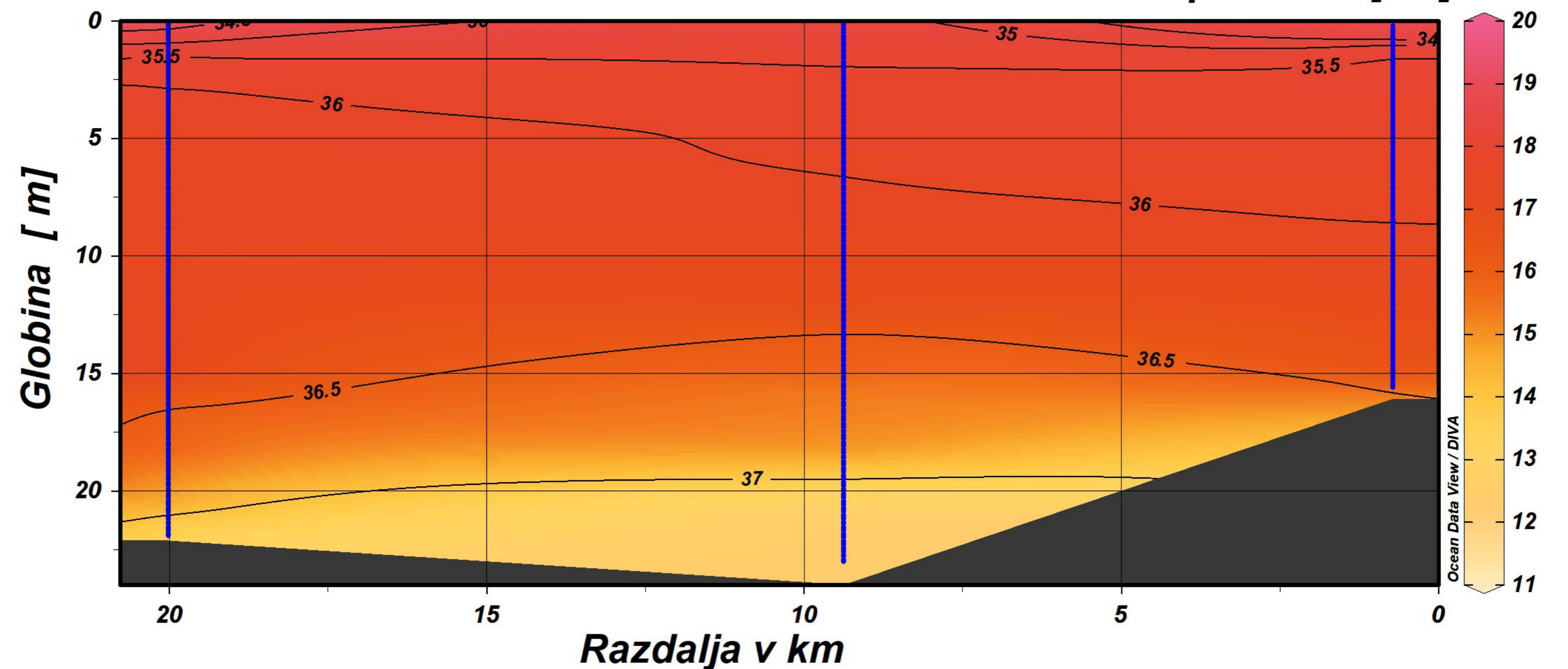
Slanost - izohaline
